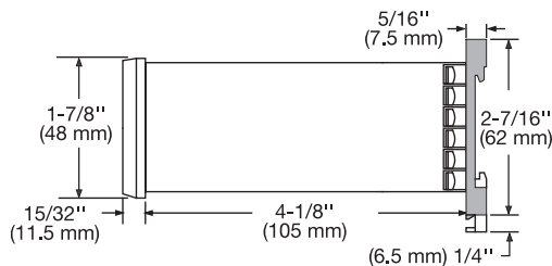
TEC-9100 DIN Rail Mount
